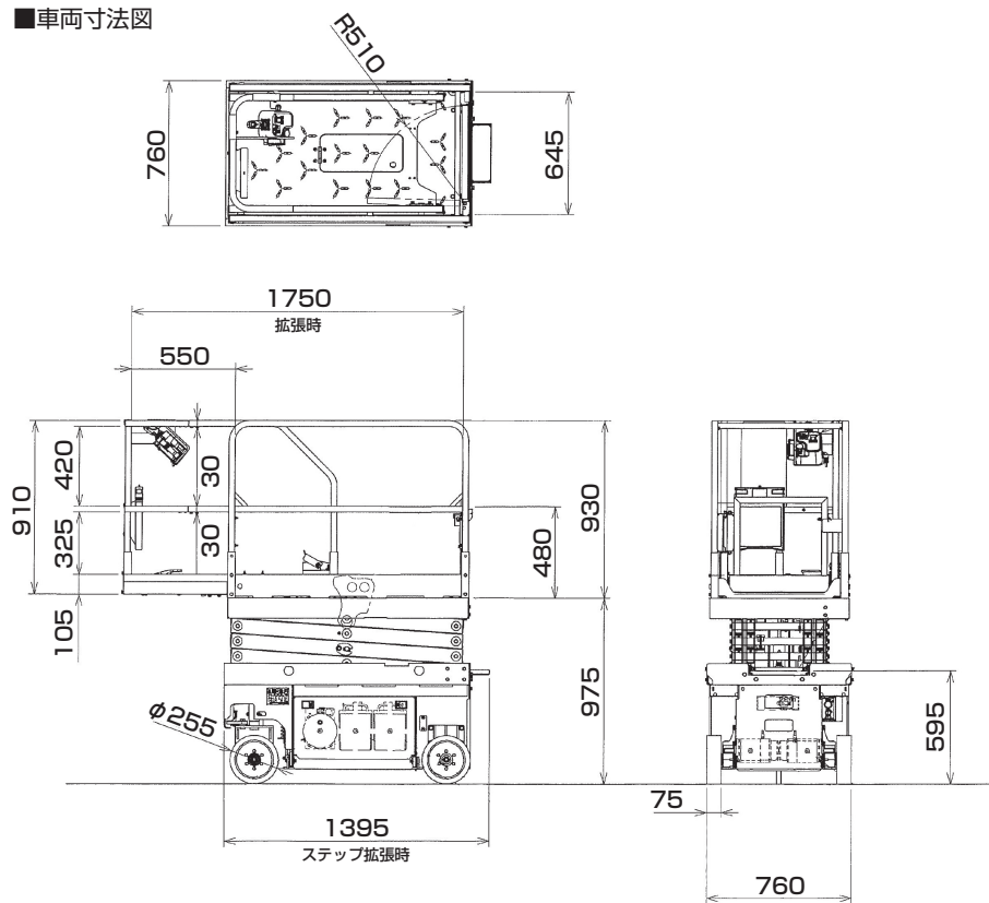
■車両寸法図
